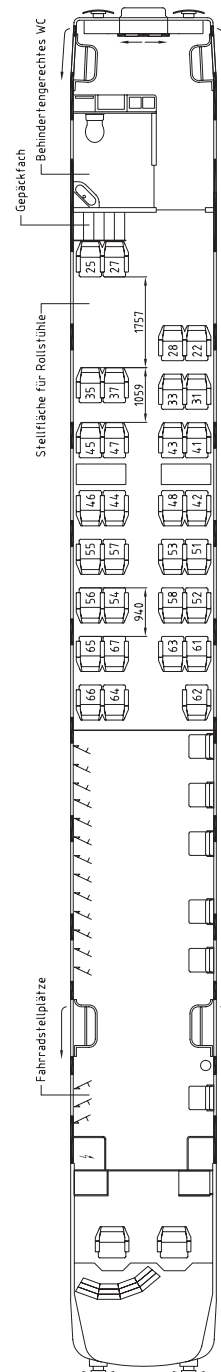
IC-Steuerwagen 2. Klasse mit 16 Fahrradstellplätzen, behindertengerecht (Bpmbdzf) Laptop-Steckdosen an den Tischen
