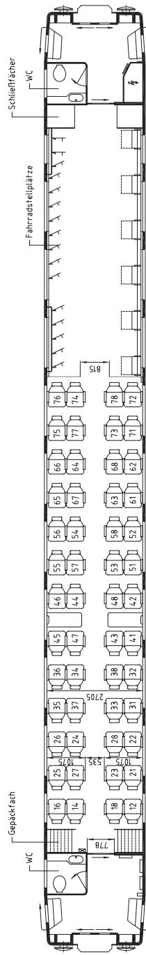
IC-Wagen 2. Klasse mit 16 Fahrradstellplätzen (Bpmd) Laptop-Steckdosen an den Tischen
