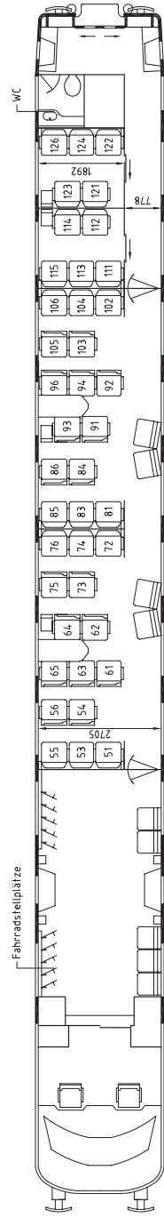
IC-Steuerwagen 2. Klasse mit 10 Fahrradstellplätzen (Bmdzf)
