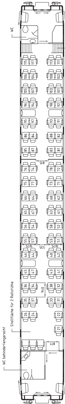
IC-Großraumwagen 2. Klasse behindertengerecht (Bpmbz) Laptop-Steckdosen an den Tischen Behinderten-WC mit Wickeltisch
