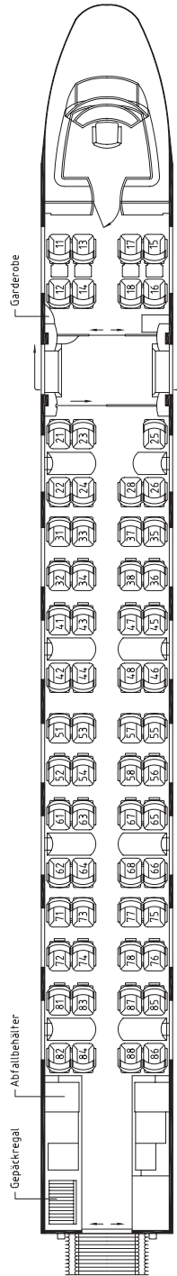
ICE TD-Endwagen 2. Klasse (Bpmpf) Wagen 27/31 Laptop-Steckdosen an allen Sitzen Lounge/Panorama Plätze 11-16
